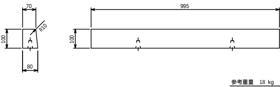
後付用水止縁石
