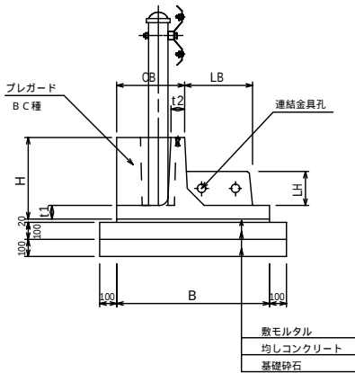
標準断面図
