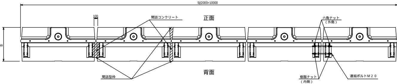
施工平面図 S = 1 : 3 0 ( 10.0m当り )
