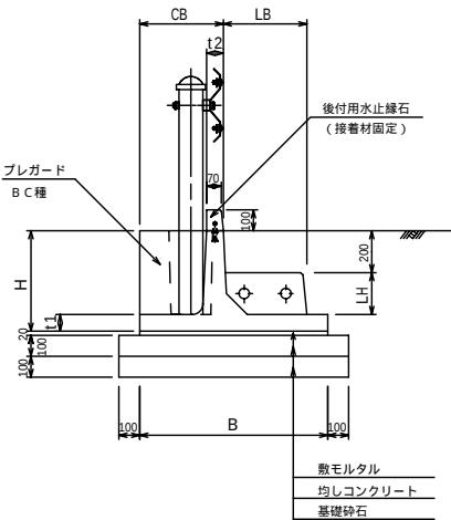
水止タイプ断面図
